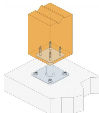
PIED REGLABLE TYPE APB REGLAGE SUR CHANTIER AVANT LA POSE
