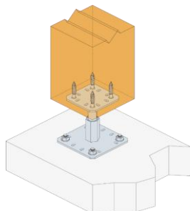
PIED REGLABLE TYPE PPRC 100 A 100 MM
