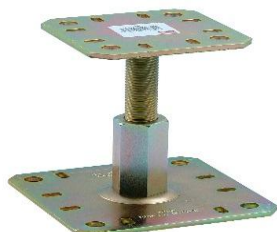
PIED REGLABLE TYPE PPRC 100 A 100 MM
