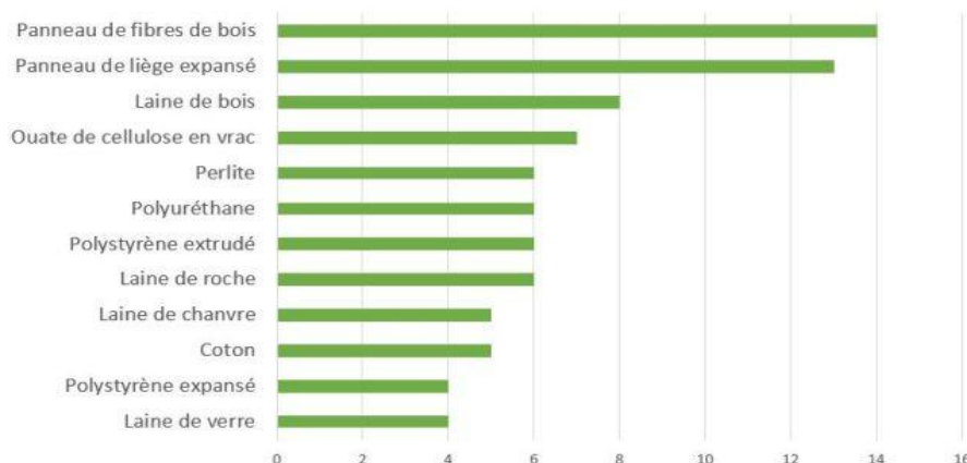
Temps de déphasage thermique (en heure)
