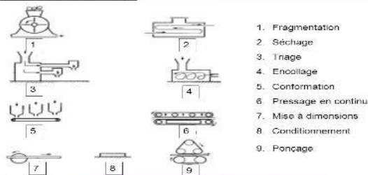
Chaîne de fabrication des panneaux agglomérés
